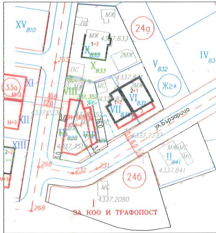
ИЗМЕНЕНИЕ НА ПЛАН ЗА РЕГУЛАЦИЯ И ЗАСТРОЯВАНЕ за УПИ VIII-351,352, ПИИ 68134.4337.351 и 68134.4337.352 кв. 24а, м. "Овча купел"
